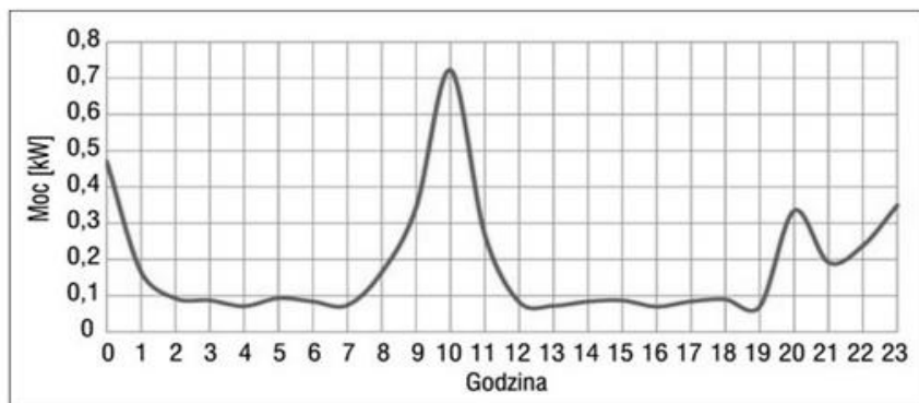
Wykres 7. Wybrany dzienny letni profil zapotrzebowania na moc w budynku jednorodzinnym
