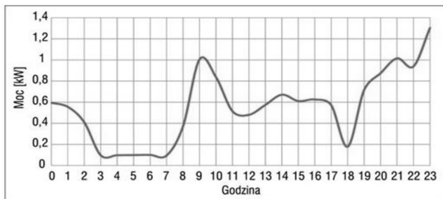
Wykres 8. Wybrany dzienny zimowy profil zapotrzebowania na moc w budynku jednorodzinnym
